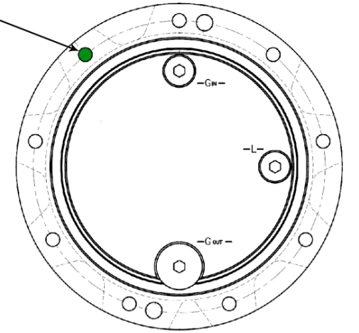
SPROCKET SIDE
